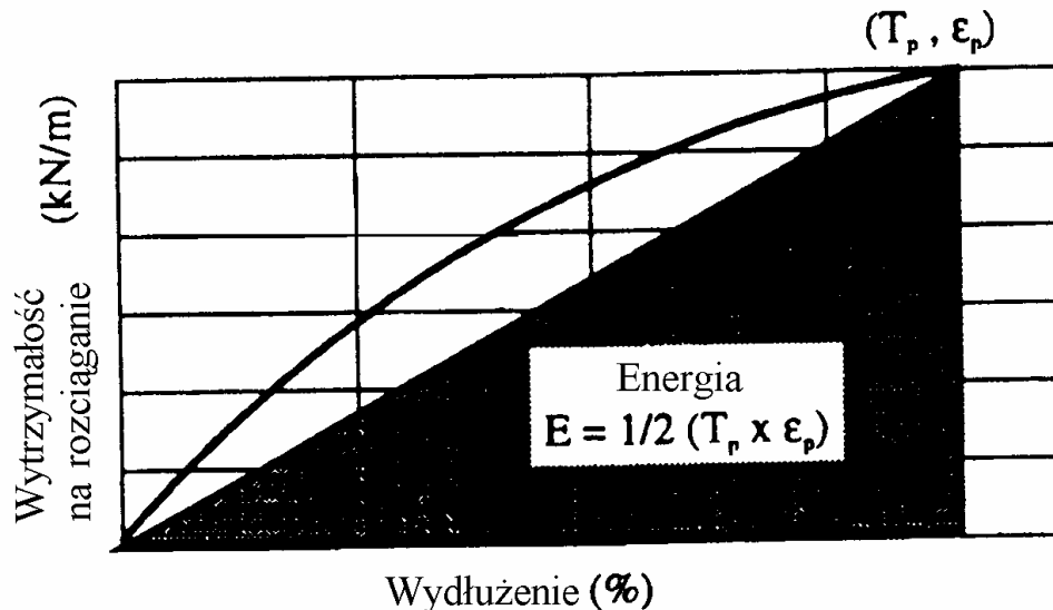
Rys. 8. Energia zniszczenia [57]
