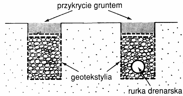
Rys. 18 Drenaż poziomy [29]
