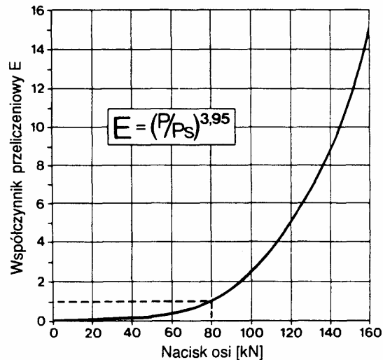
Rys. 28 Nomogram do przeliczenia obciążenia na osie standardowe
