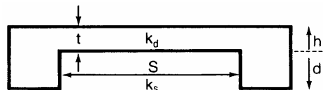
Rys. 39. Schemat do obliczenia grubości poziomej warstwy drenującej [29]
