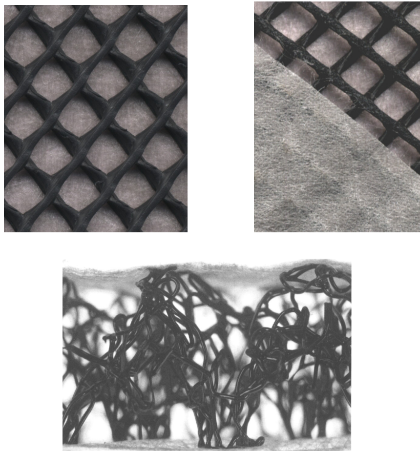
Rys. 4. Przykłady geokompozytów
