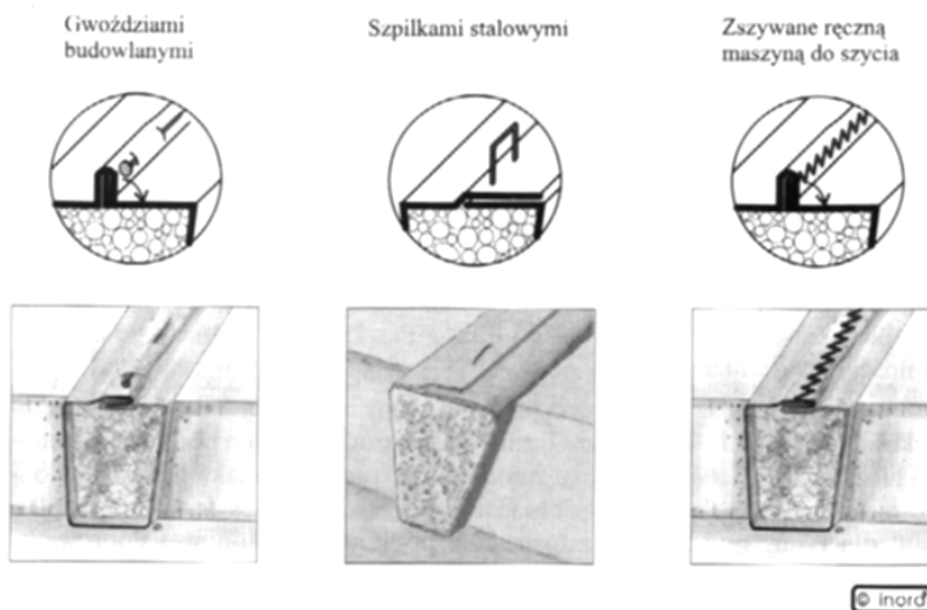
Rys. 25. Przykładowe sposoby zamykania drenu francuskiego [25]
