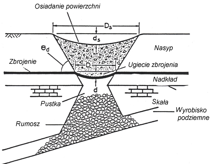
Rys. 17. Działanie zbrojenia z geotekstyliów w nasypie na podłożu zapadliškowym
